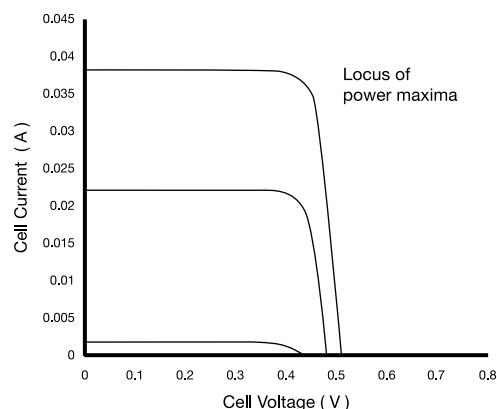
Fig. 1 – Thycon MPPT
